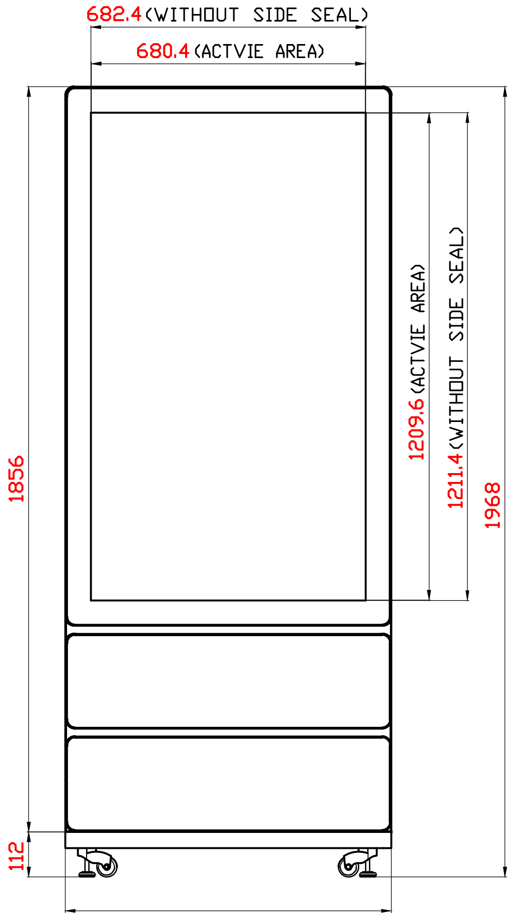
正視圖
