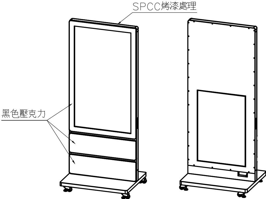
正面 Scale 1:2
