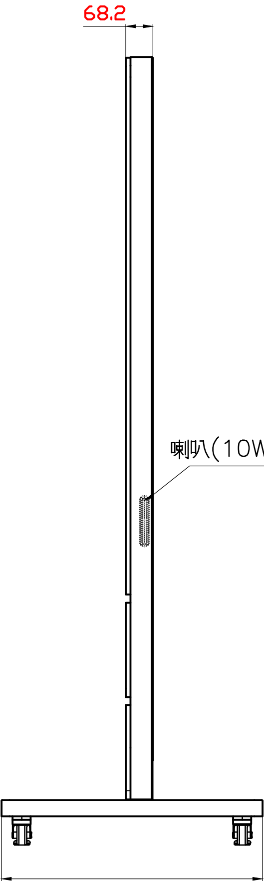
右側視圖
