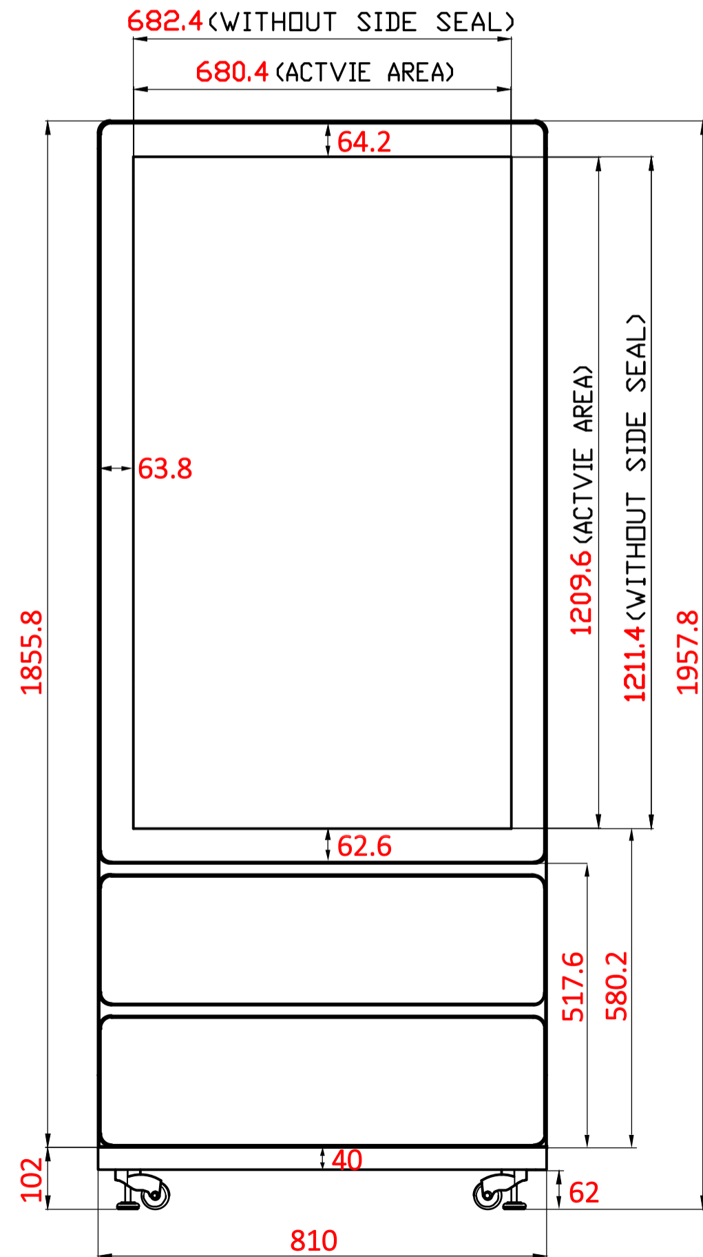
正視圖
