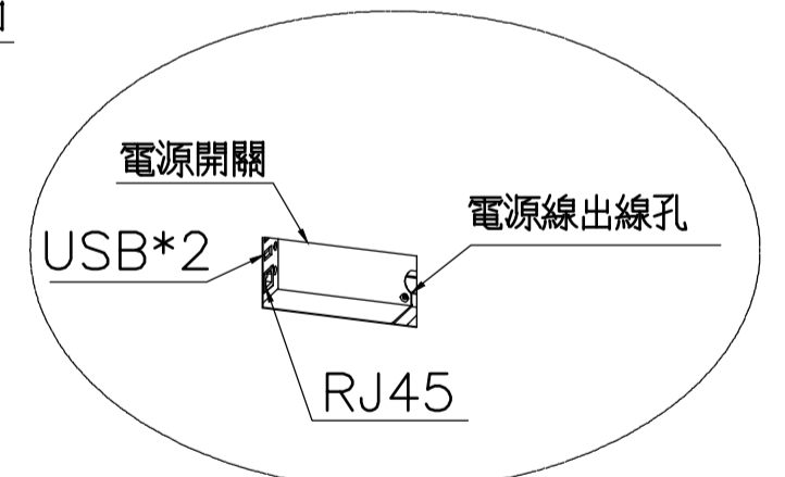
視圖P
