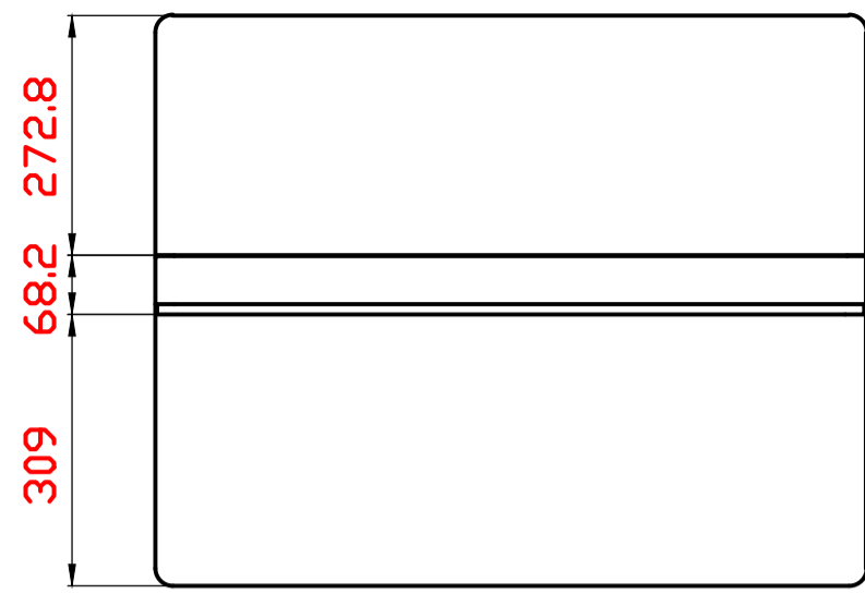
上視圖
