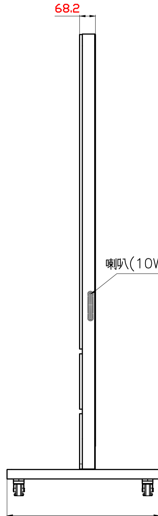
右側視圖
